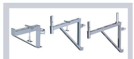
Konsol 300, 700, 800 Nyckelvidd 22 mm Fzv
