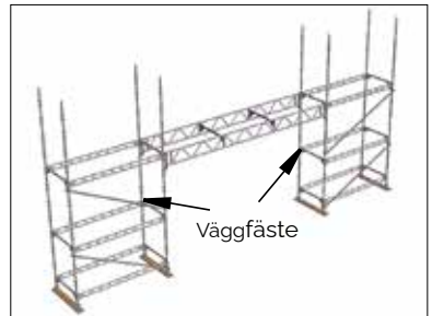
Fackverksbalk i aluminium
